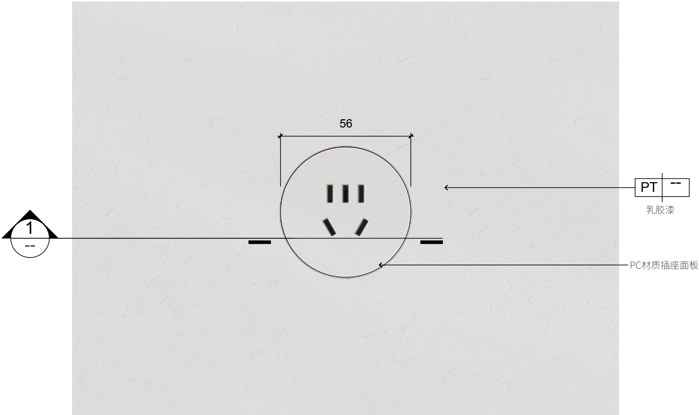
PLAN 墙面插座平面图 SCALE: 1:1.7
