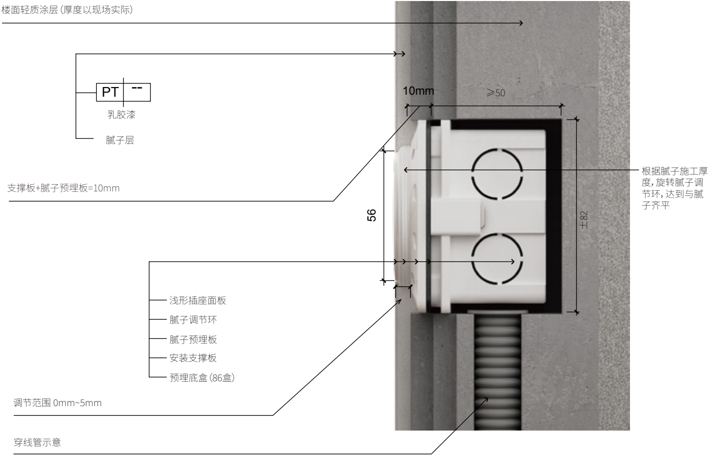
DETAIL 墙面插座剖视图 SCALE: 1:1.7
