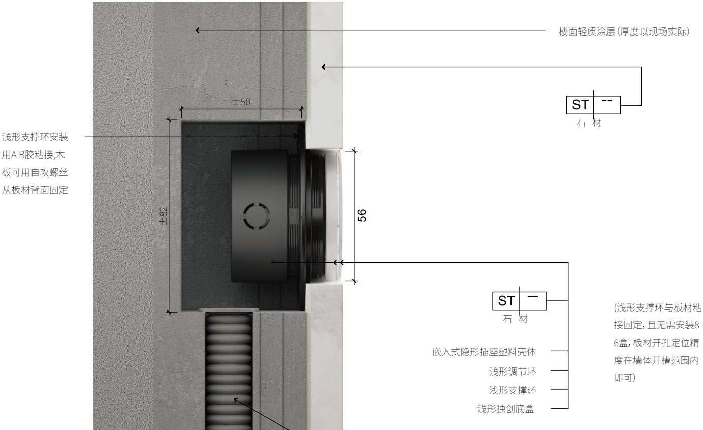
DETAIL 石板面插座剖面图 SCALE: 1:1.7
